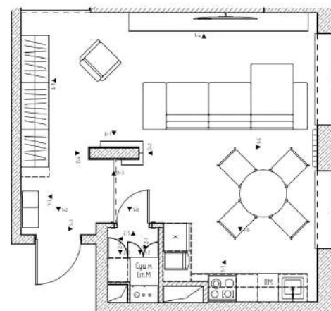
Фрагмент плана с развертками 180
