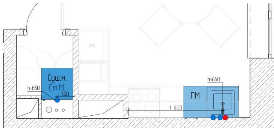
Фрагмент плана сантехники М1:30
