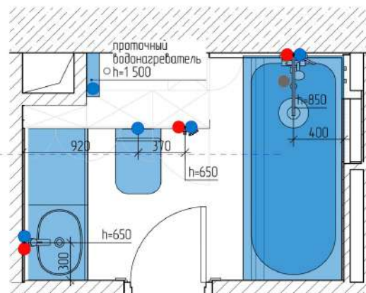
Фрагмент плана сантехники М1:30
