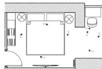
Фрагмент плана с развертками 180
